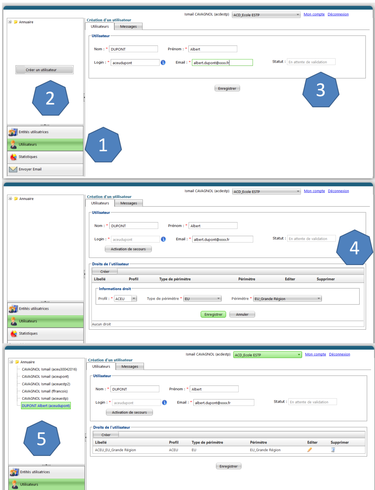
Figure 13 – Création d'un profil ACEU
